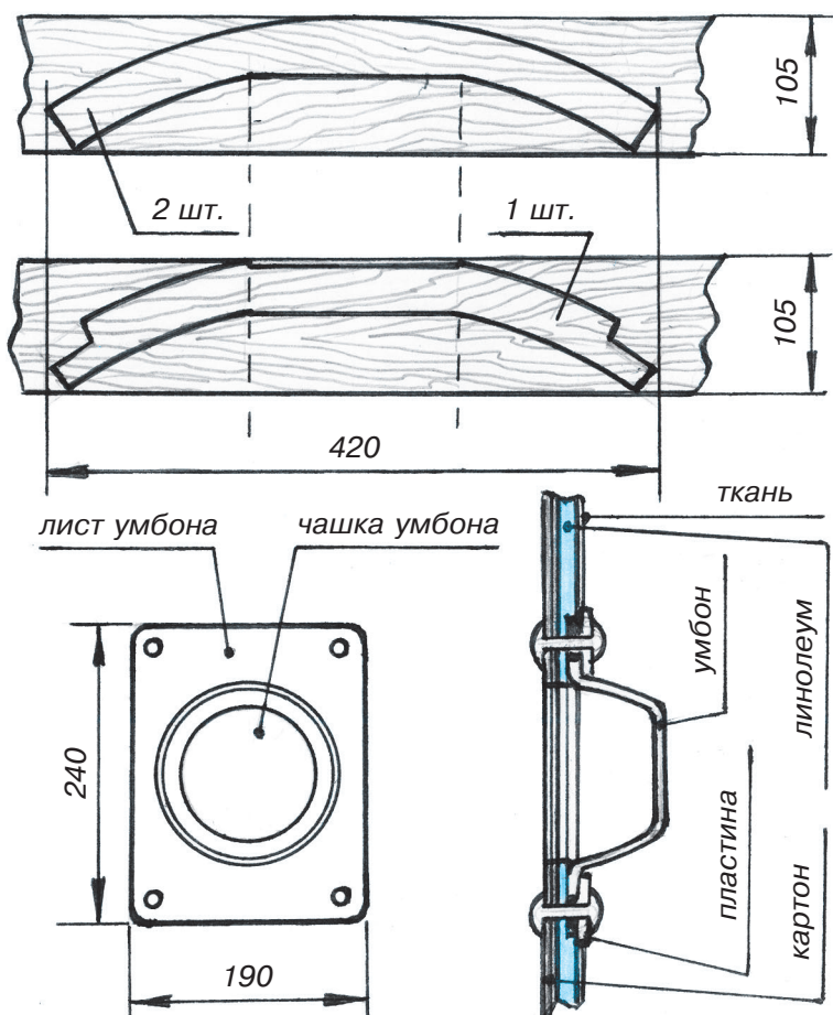
Рис. 2. Детали скутума.
