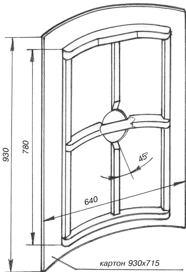
Рис. 1. Каркас щита.
